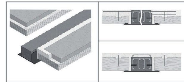
Holz-Beton-Verbunddecken (Betonfertigteilprofil). Holzplatten.
