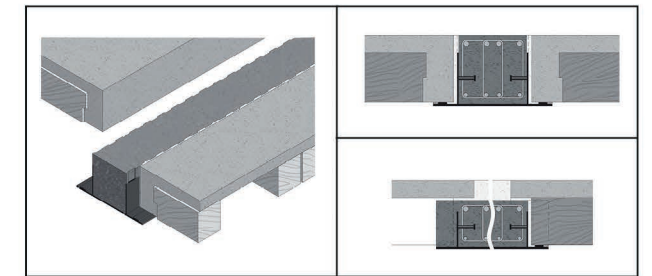
Holz-Beton-Verbunddecken (Betonfertigteil). Rippen aus Holz.
