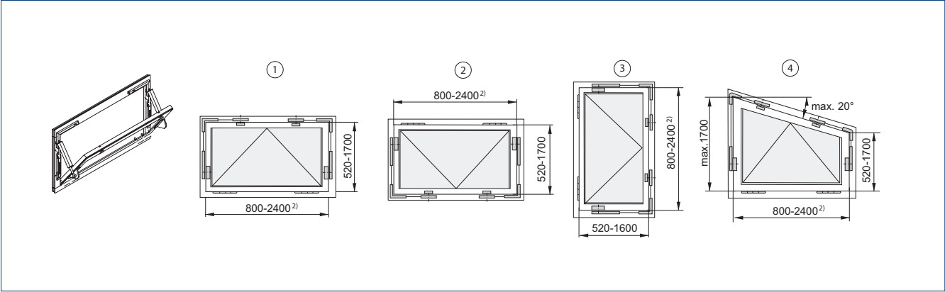
Alle Angaben in mm 1 = Kippfenster | 2 = Klappfenster | 3 = Drehfenster | 4 = Schrägfenster | 2) Für Kunststofffenster Syncro max. 1600 mm
