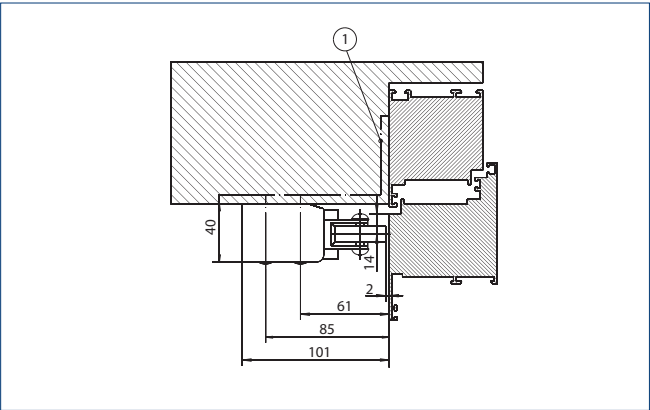
Detail Kopfpunkt
