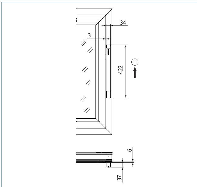
Platzbedarf Rahmenmontage
