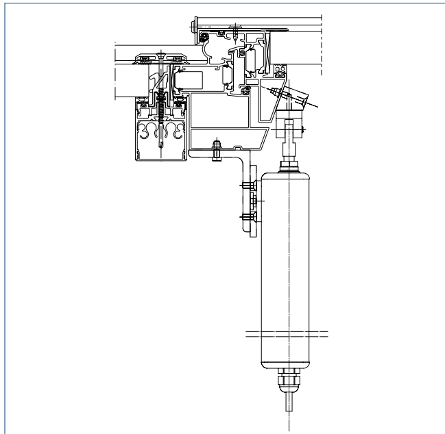
Adapter für Konsole E 250 NSK S (Id.Nr. 138370) | Drehkonsole E 250 NT + E 350 N (Id.Nr. 116112) | Winkel E 250 NSK (Id.Nr. 138369)
