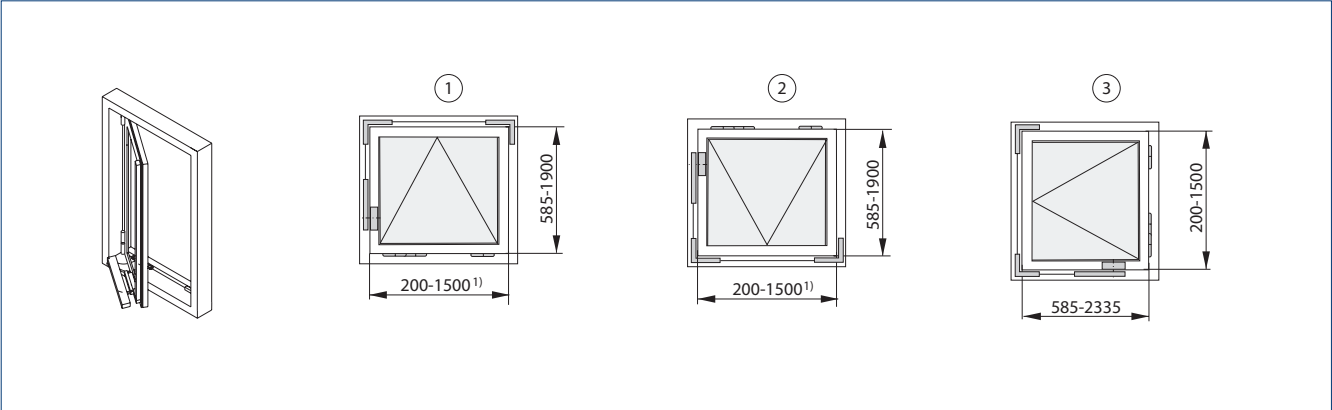
Alle Angaben in mm 1 = Kippfenster | 2 = Klappfenster | 3 = Drehfenster | 1) Für Kunststofffenster Solo max. 800 mm
