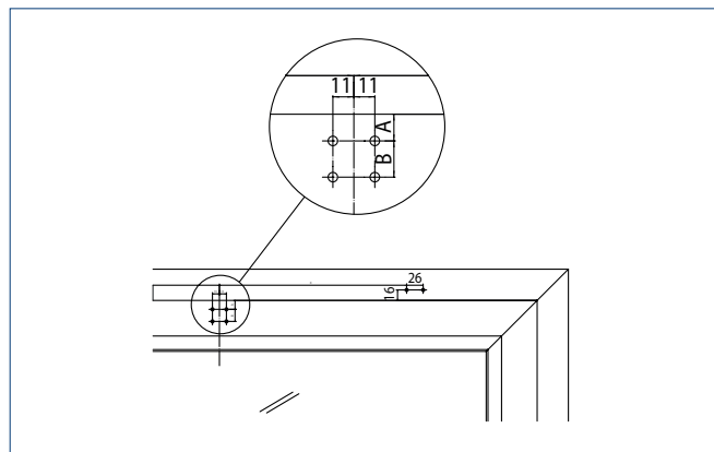
Rahmenmontage EINWÄRTS
