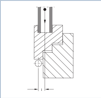
i = Abstandmaß vom Flügelschwerpunkt zum Banddrehpunkt [mm]
