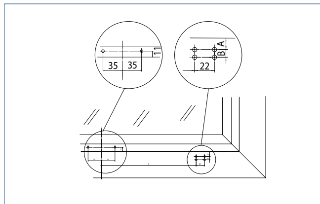
Flügelmontage EINWÄRTS
