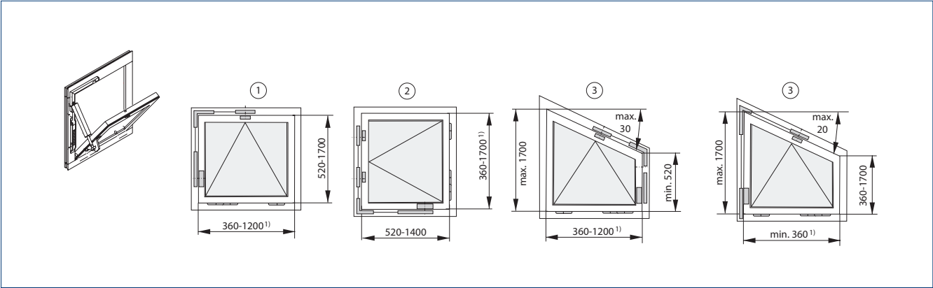
Alle Angaben in mm 1 = Kippfenster | 2 = Drehfenster | 3 = Schrägfenster Kipp | 1) Für Kunststofffenster Solo max. 800 mm
