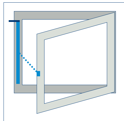
Drehflügel DIN R EINWÄRTS (Antrieb nicht schwenkbar) Kabelaustritt immer nach oben!
