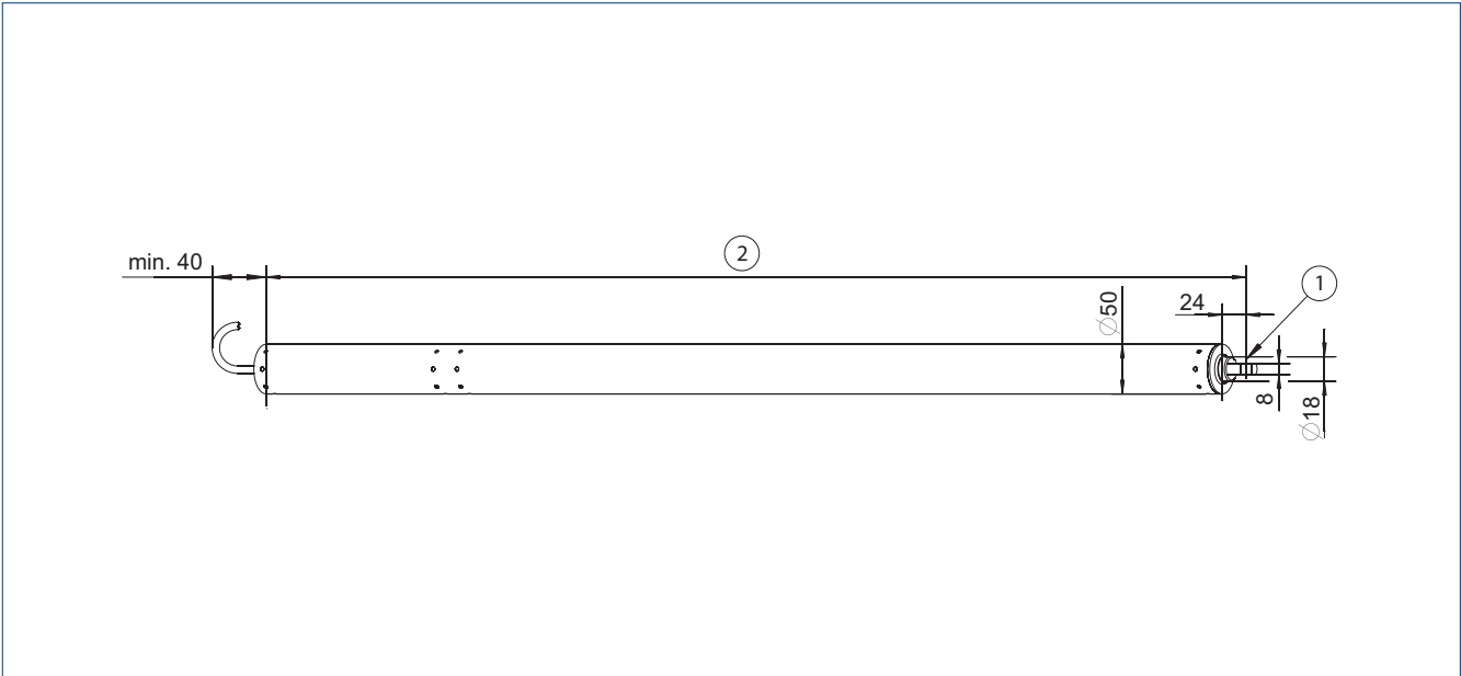
1 = ø 6 mm mit Lagerbuchse, ø 8 mm ohne Lagerbuchse | 2 = ca. 465 mm + Hub
