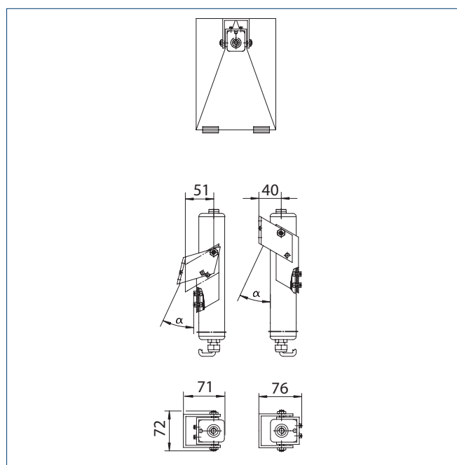
Standardkonsole
