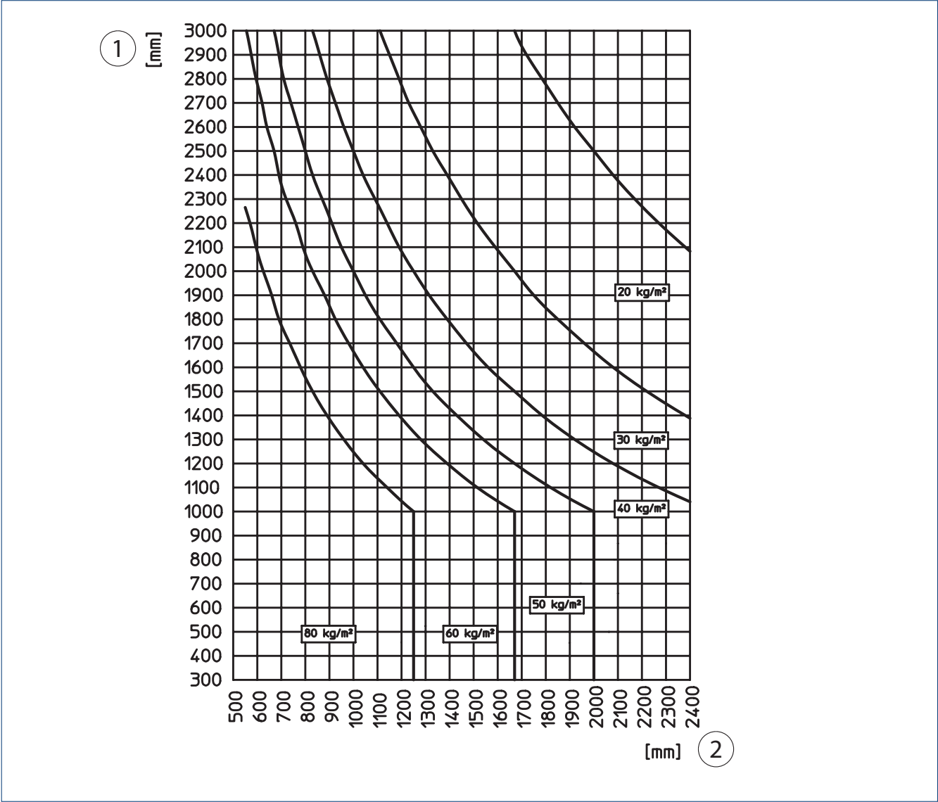
1 = Flügelhöhe | 2 = Flügelbreite
