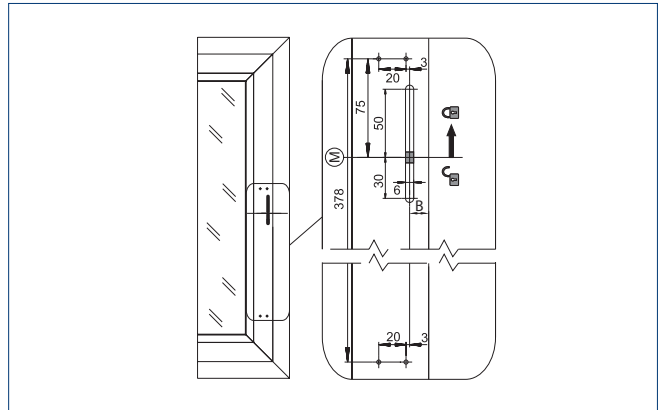
Montagemasse Flügelmontage
