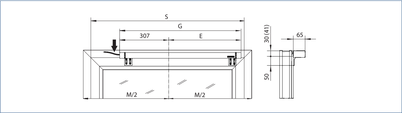
Maße für E, G und S siehe Tabelle Maß in Klammern gilt für Drehfenster DIN rechts
