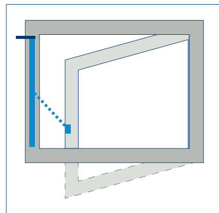
Drehflügel DIN L AUSWÄRTS (Antrieb nicht schwenkbar) Kabelaustritt immer nach oben!
