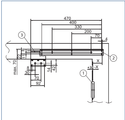
Montage Konsolen
