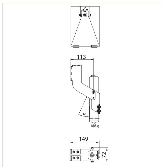
Konsole EINWÄRTS
