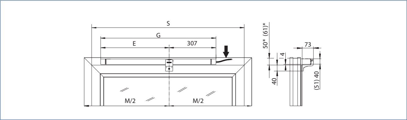
Maße für E, G und S siehe Tabelle Maße in Klammern gelten für Drehfenster DIN links | * = Schwenkbereich
