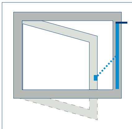
Drehflügel DIN R AUSWÄRTS (Antrieb nicht schwenkbar) Kabelaustritt immer nach oben!
