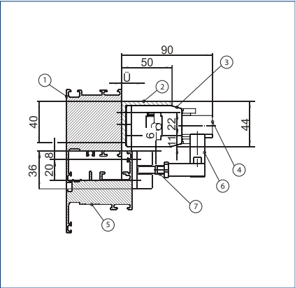
Detail Kopfpunkt
