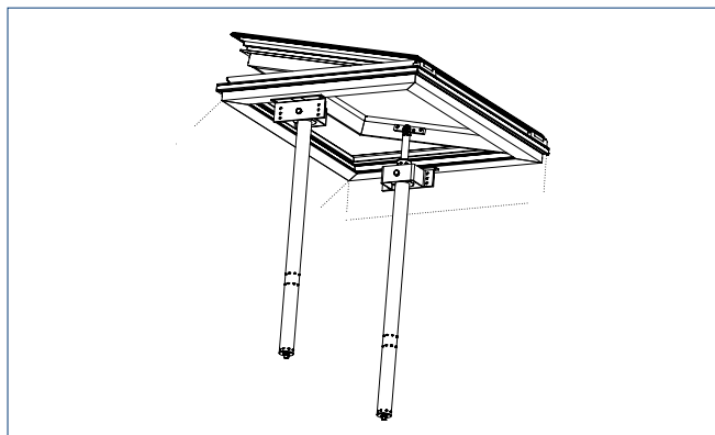
Nebenschließkantenmontage Syncro
