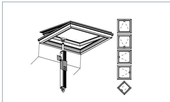
Standardkonsole für Montage am Sturz der Hauptschließkante
