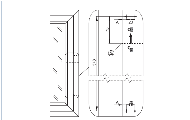
Montagemasse Rahmenmontage
