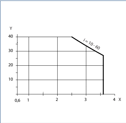
X = Gesamtflügelbreite (Summe aller Flügelbreiten) [m] | Y = Füllgewicht [kg/m²]
