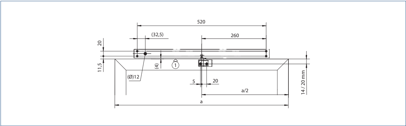
1 = Oberkante Flügel
