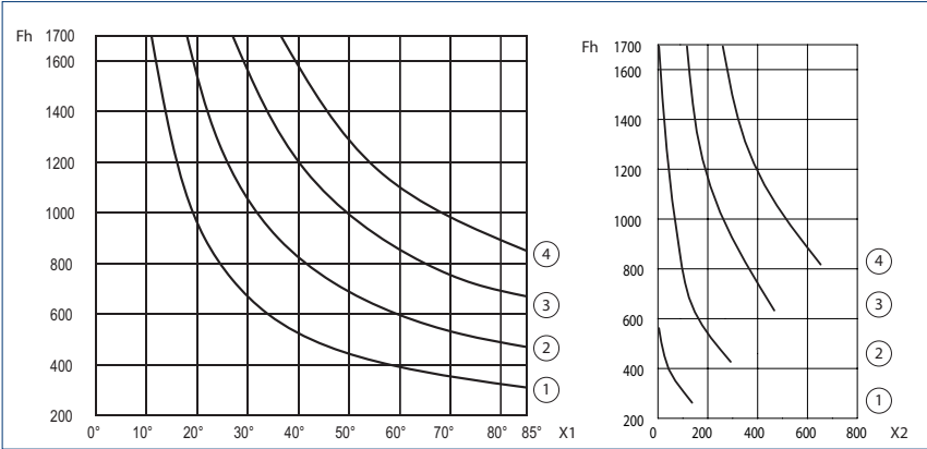
X1 = Öffnungswinkel | X2 = Platzbedarf für Schwenkung (mm) | Fh = Flügelhöhe (mm) | 1 = Hub 300 | 2 = Hub 500 | 3 = Hub 750 | 4 = Hub 1000
