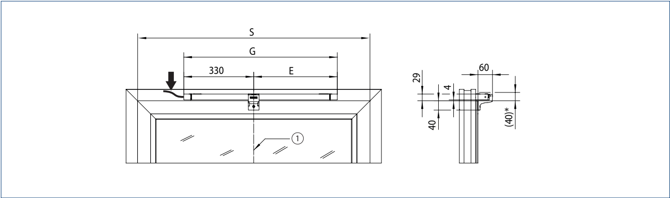
Maße für E, G und S siehe Tabelle 1 = Mitte Fenster | * = Schwenkbereich
