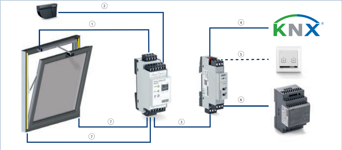
1 = Anschlusskabel Antrieb A/B/S/L (4-adrig) | 2 = Sensor GC 342, angebracht an der Fensterausßenseite +24 V / GND / TST /Si | 3 = Verbindungskabel IQ box Safety und IQ box KNX A/B/S/L (4-adrig) | 4 = KNX Bus (2-adrig) | 5 = Lüftertaster (optional) | 6 = Netzteil 24 V / GND (2-adrig) | 7 = Anschluss Schaltleiste
