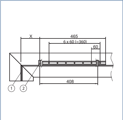
Montage Gleitschiene
