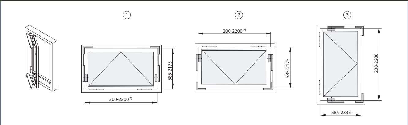
Alle Angaben in mm 1 = Kippfenster | 2 = Klappfenster | 3 = Drehfenster | 1) Für Kunststofffenster Syncro max. 1600 mm
