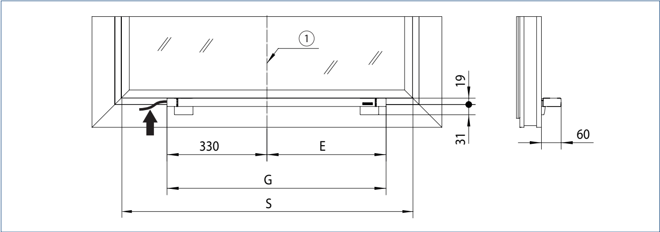
Maße für E, G und S siehe Tabelle 1 = Mitte Fenster
