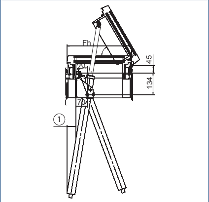
Fh = Flügelhöhe | 1 = Freier Platz unter dem Fenster für die Schwenkbewegung des Antriebs während der Öffnungsbewegung, siehe Diagramm
