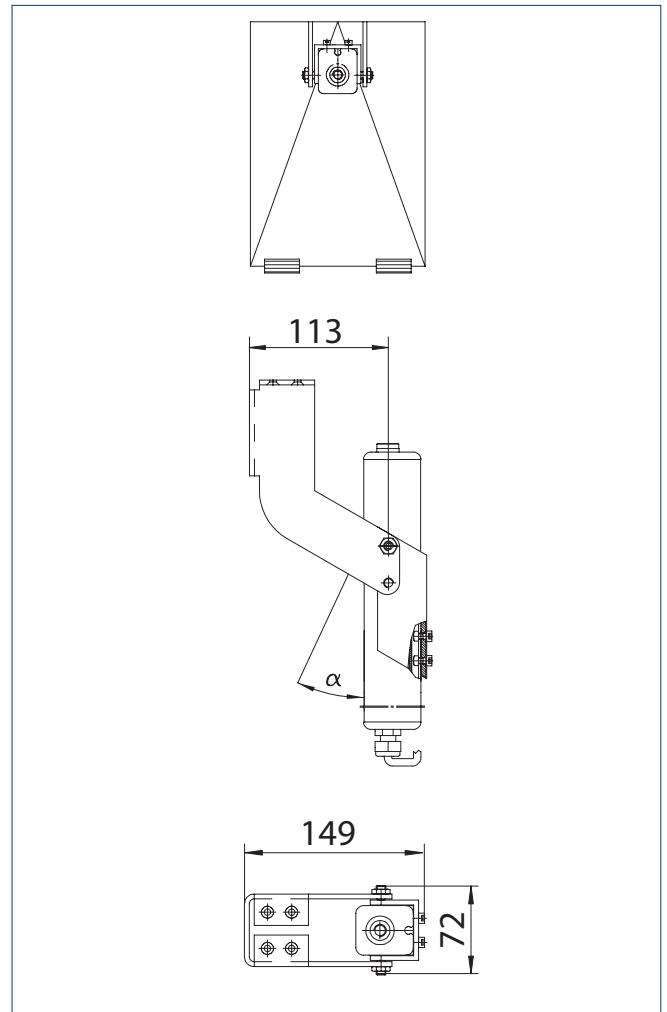
Konsole EINWÄRTS
