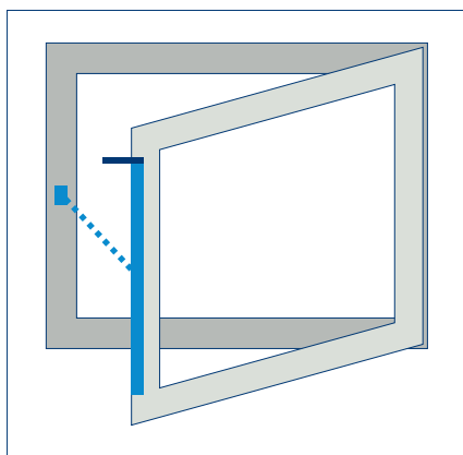
Drehflügel DIN R EINWÄRTS (Antrieb nicht schwenkbar) Kabelaustritt immer nach oben!
