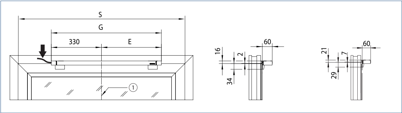
Maße für E, G und S siehe Tabelle 1 = Mitte Fenster
