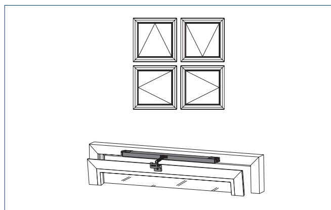
Konsolensatz A
