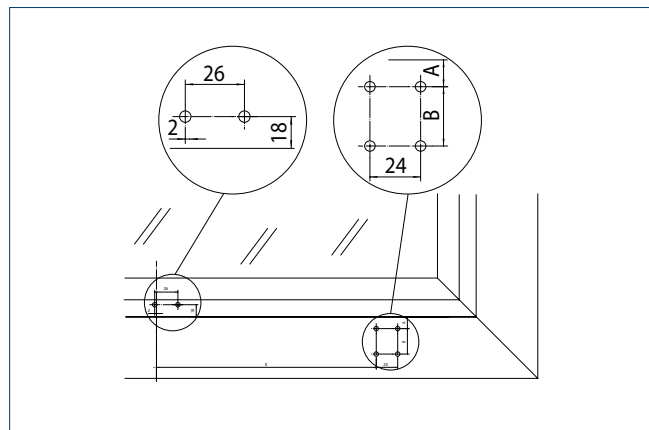
Flügelmontage EINWÄRTS
