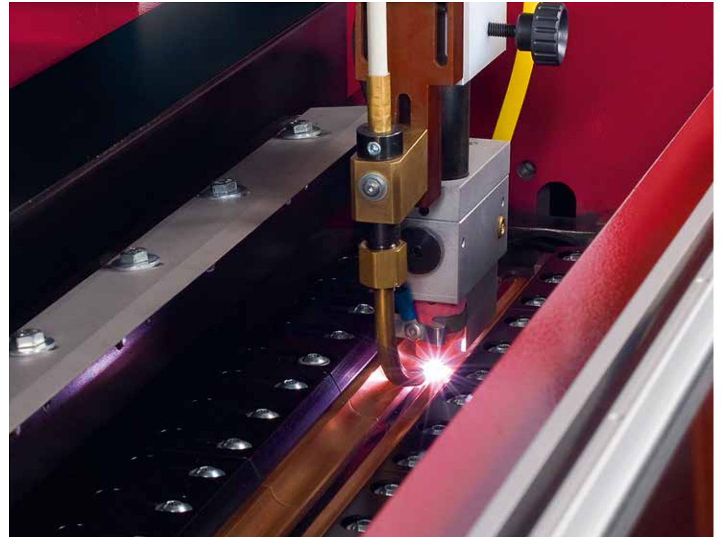
PLASMA-LÄNGSSCHWEISSEN
